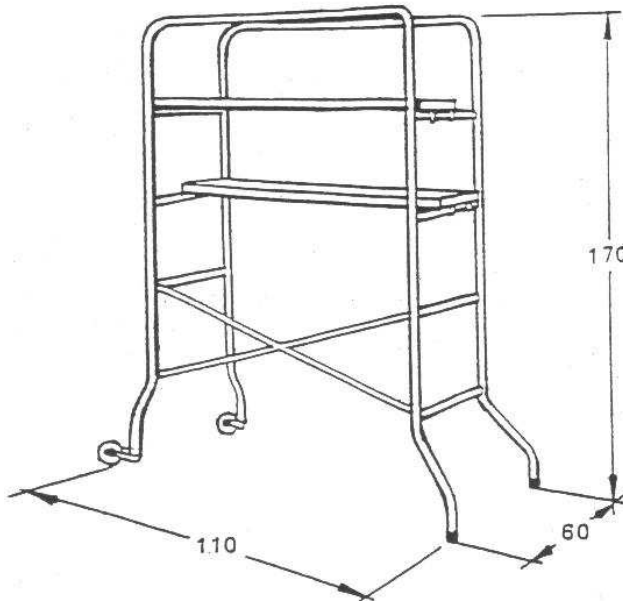
Art. 434 PONTEGGIO in acciaio da mt. 1,70 altezza x 110x0,60 trasformabile in Scala da mt. 3
